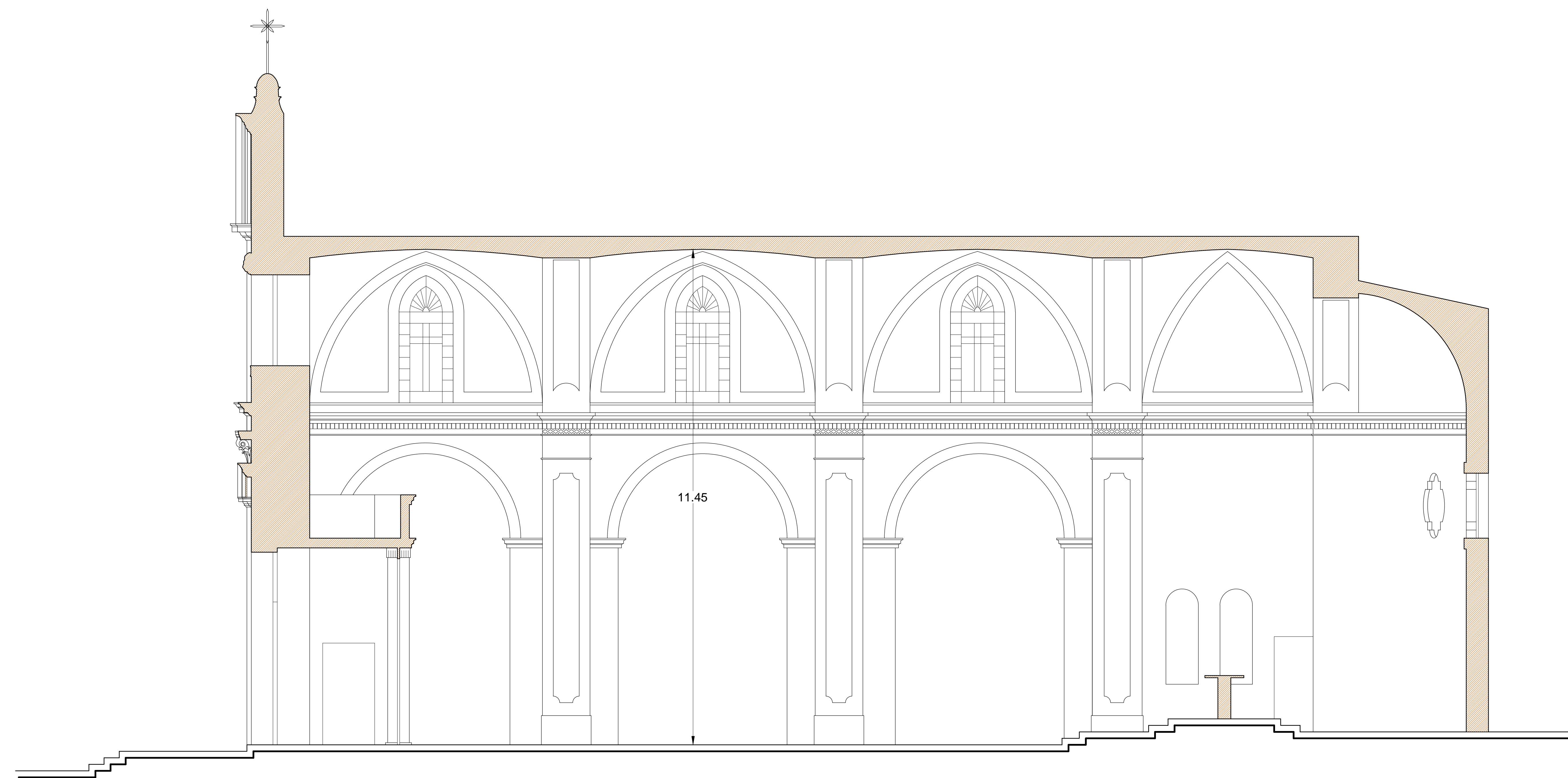
SEZIONE B-B
