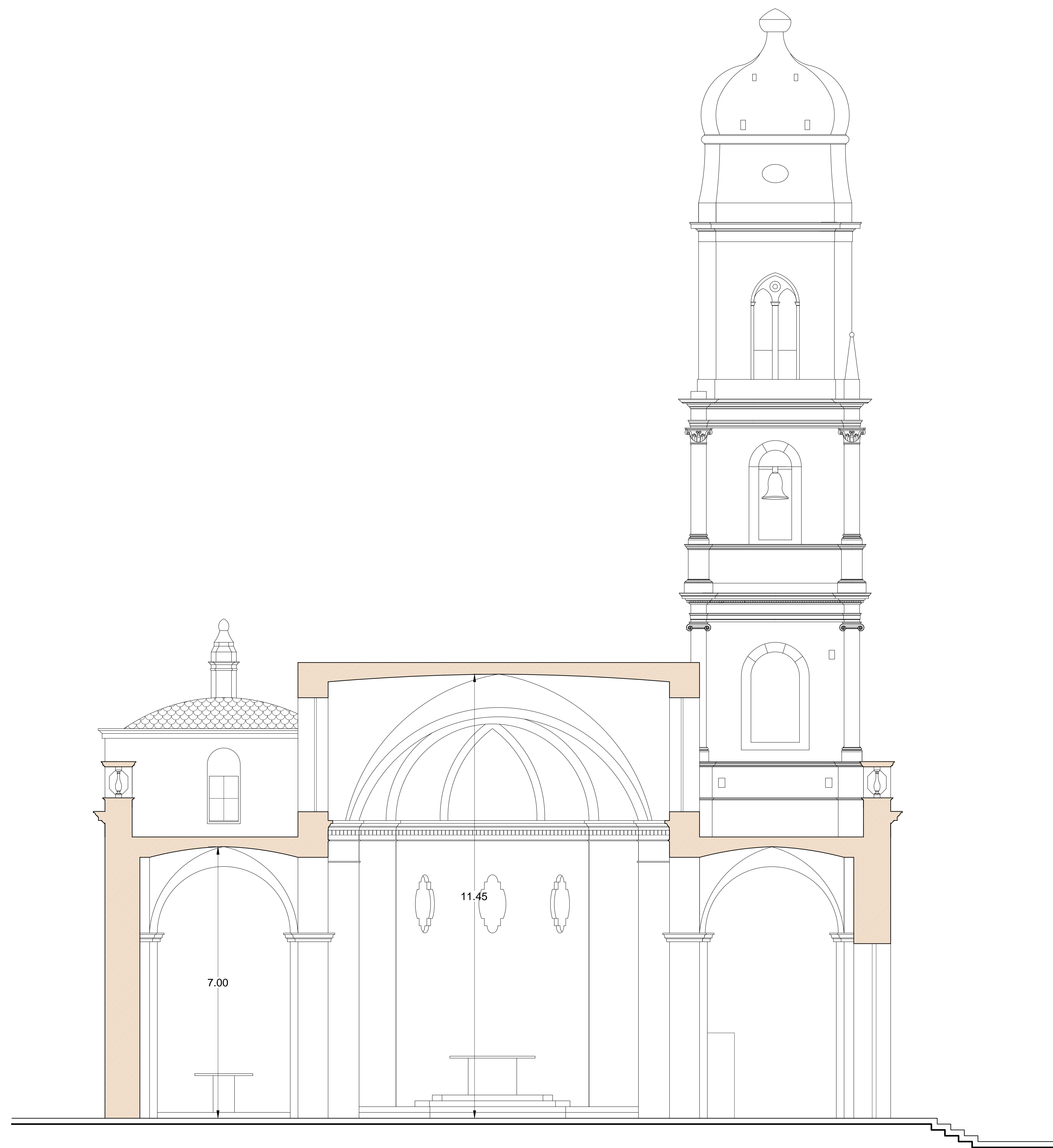
SEZIONE A-A
